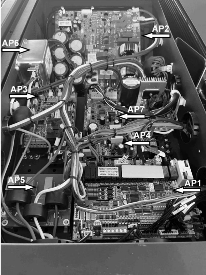
Abb. 81: E-Kasten ecoWP 2Xe 18
