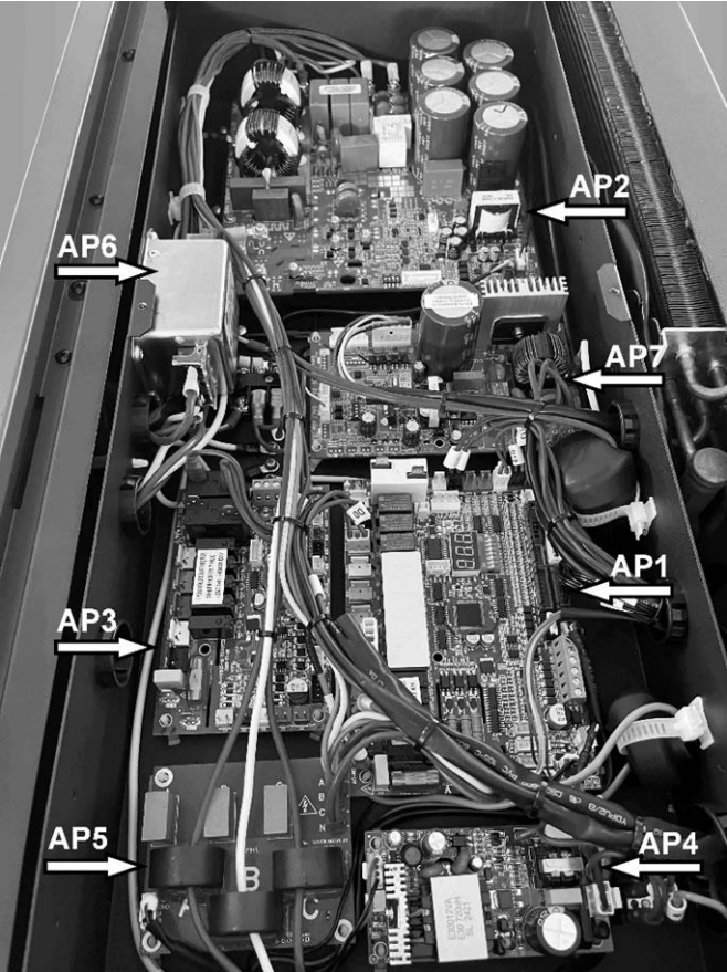
Abb. 4: E-Kasten ecoWP 2Xe 8 und 12
