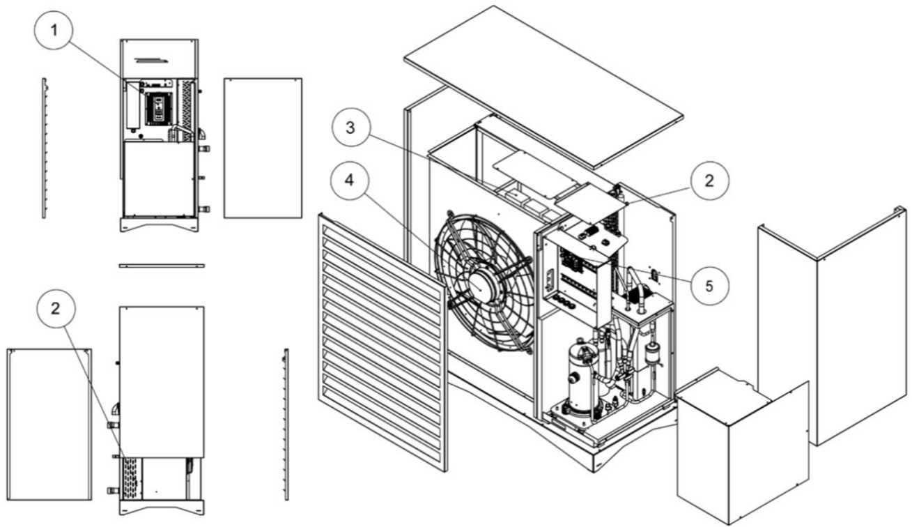
Abb. 43: Komponenten Außeneinheit
