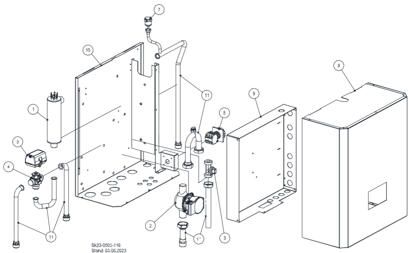
Abb. 45: Regelungseinheit ecoWP Xe
