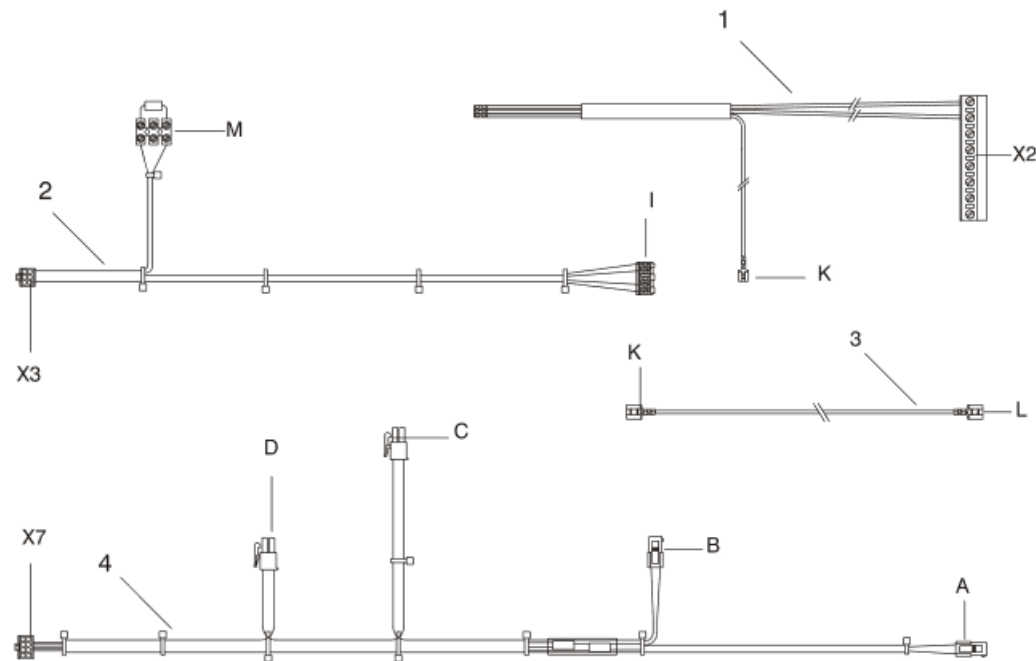
Abb. 162: Verdrahtung
