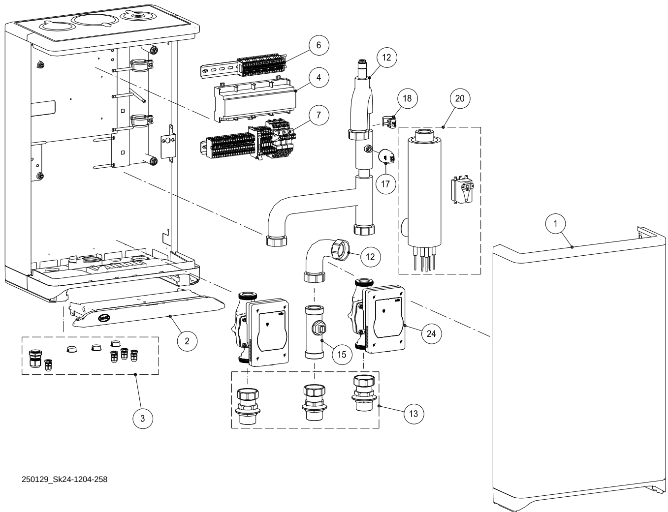
Abb. 8: Regelungseinheit ecoWP 2Xe 12 und 18
