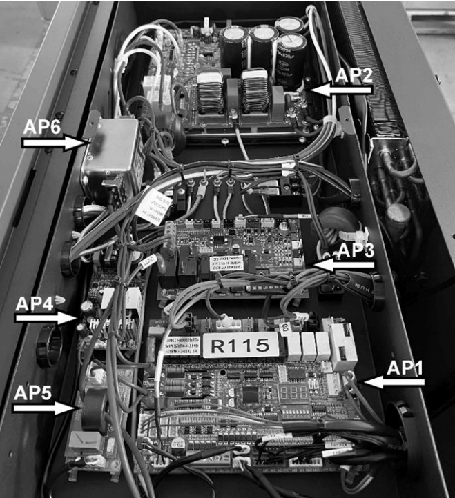
Abb. 3: E-Kasten ecoWP 2Xe 6
