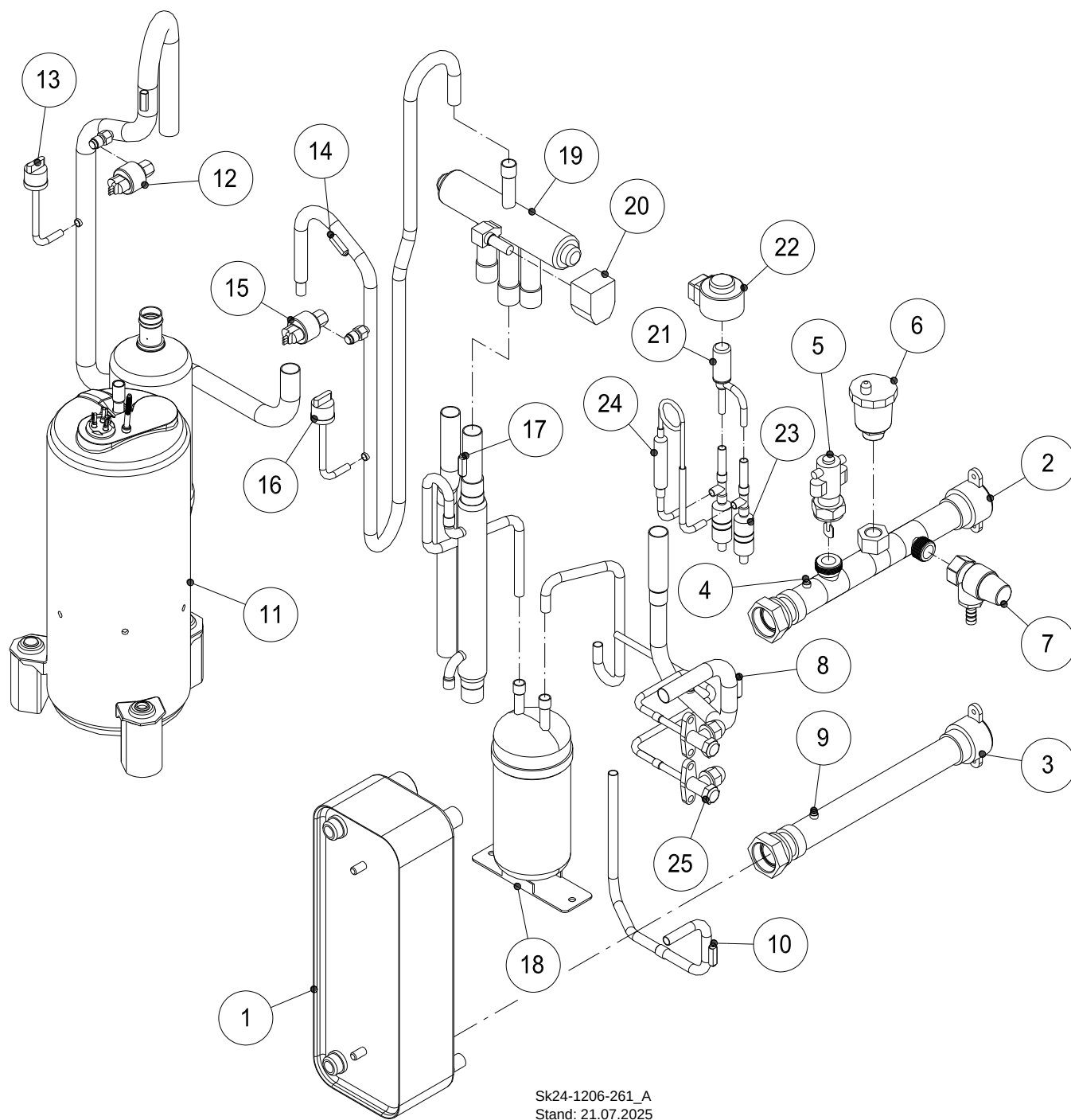
Abb. 5: Kältekreis Außeneinheit ecoWP 2Xe 6, 8 und 12
