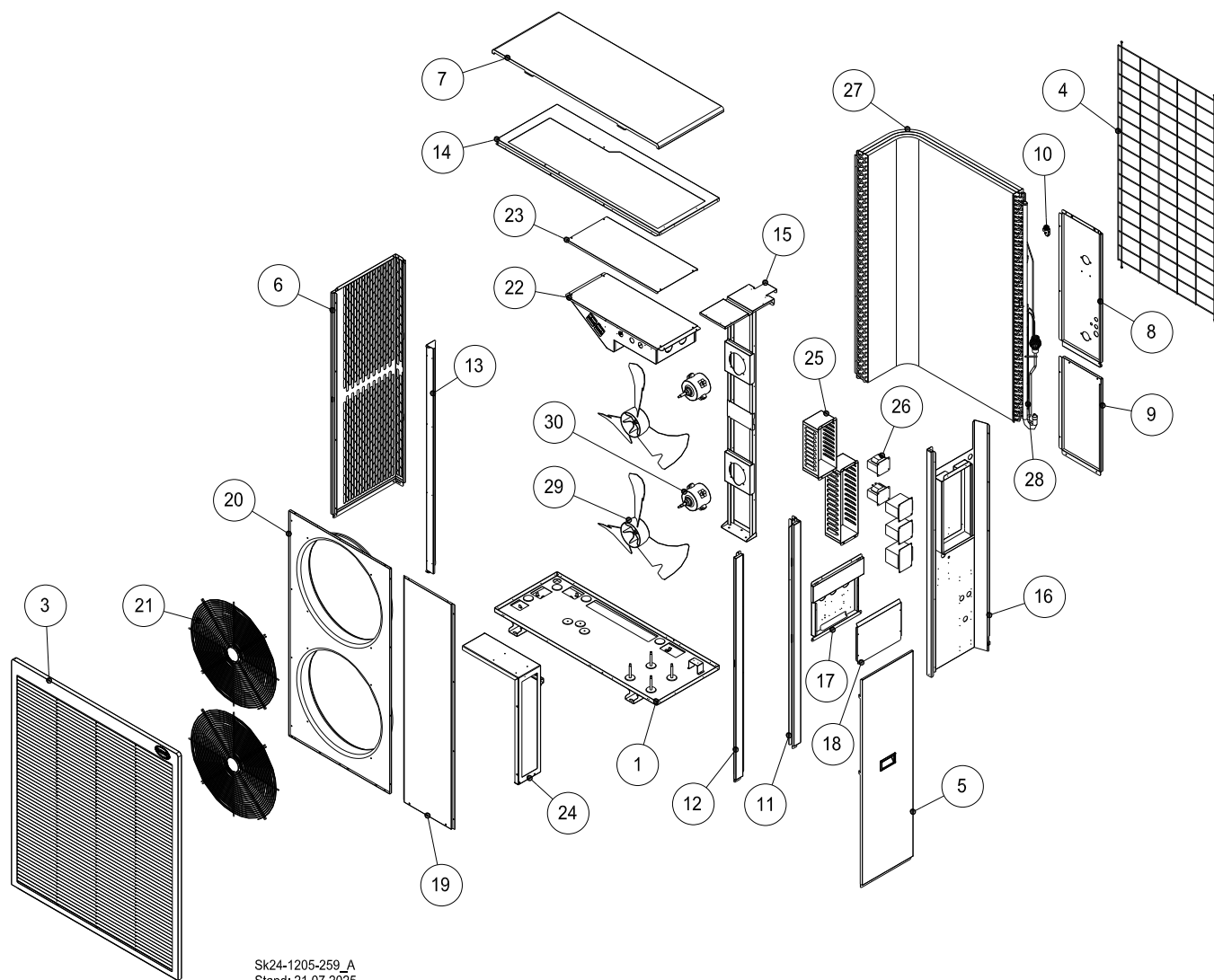
Abb. 2: Gehäuse und Komponenten Außeneinheit ecoWP 2Xe 18
