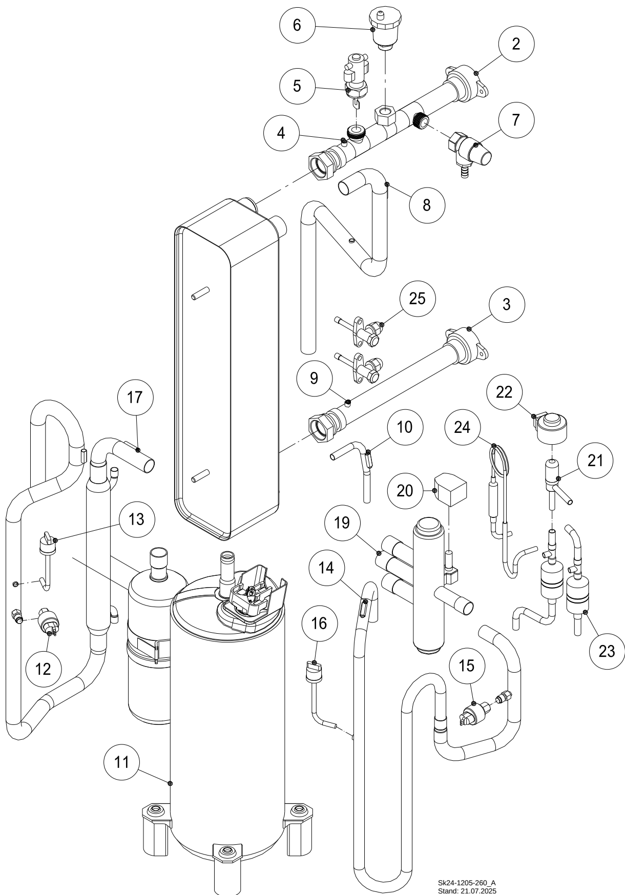
Abb. 6: Kältekreis Außeneinheit ecoWP 2Xe 18
