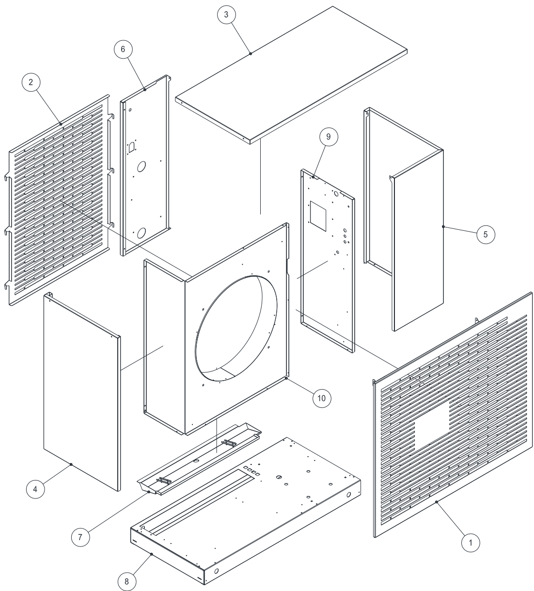
Abb. 42: Gehäuse Außeneinheit
