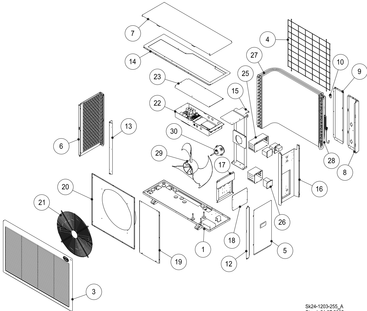
Abb. 1: Gehäuse und Komponenten Außeneinheit ecoWP 2Xe 6, 8 und 12
