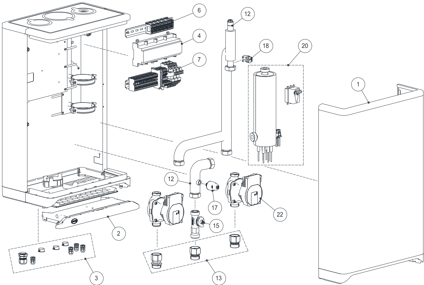
Abb. 7: Regelungseinheit ecoWP 2Xe 6 und 8
