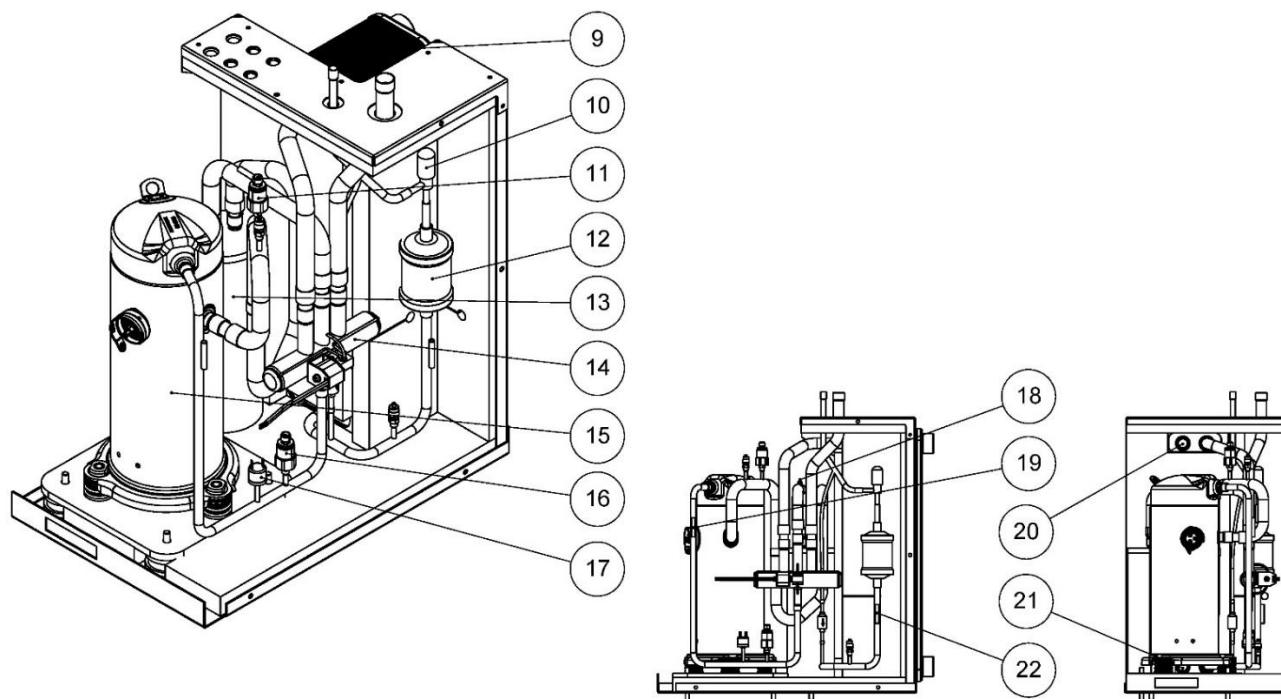
Abb. 9: Kältekreis Außeneinheit
