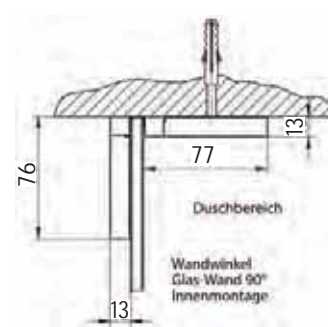
Wandwinkel nach innen
