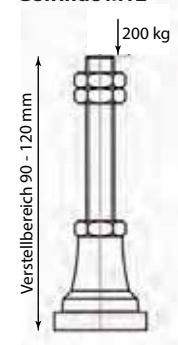
Wannenfuß Gewinde M12
