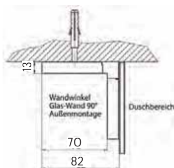
Wandwinkel nach außen
