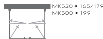
U-Kabine mit Drehfalttür 4-teilig mit Festteilen
