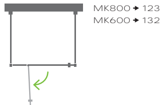
Drehtür mit Festteil und zwei Seitenwänden
