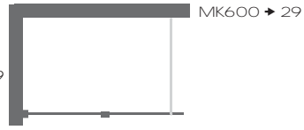
Duschwand senkrecht geteilt
