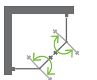
Fünfeckdusche mit Pendeltür
