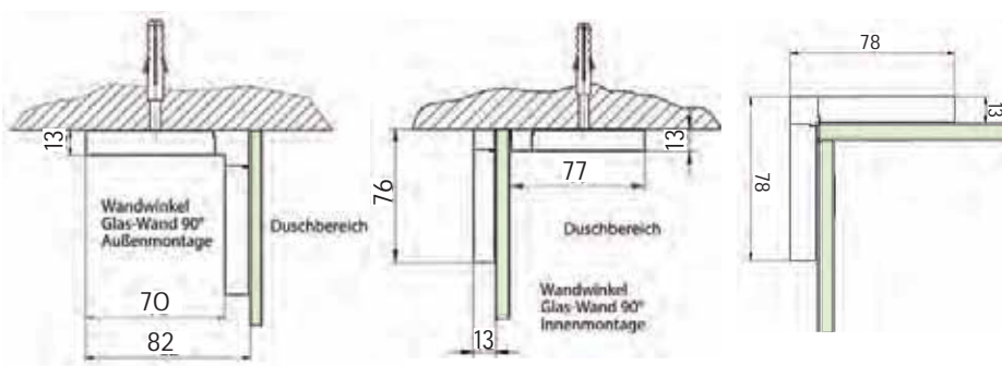
Wandwinkel nach außen
