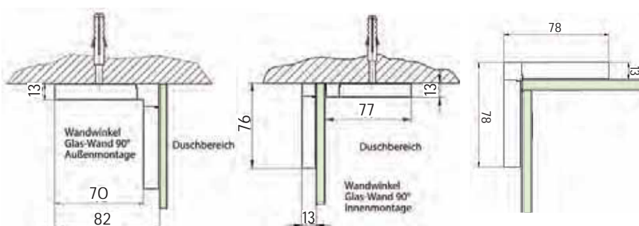
Wandwinkel nach außen
