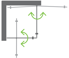
Eckeinstieg Drehtür 4-teilig/2-teilig
