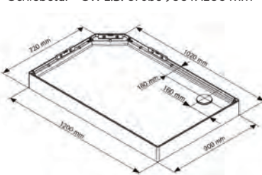
Schiebetür + SW z.B. Größe 900 x 1200 mm
