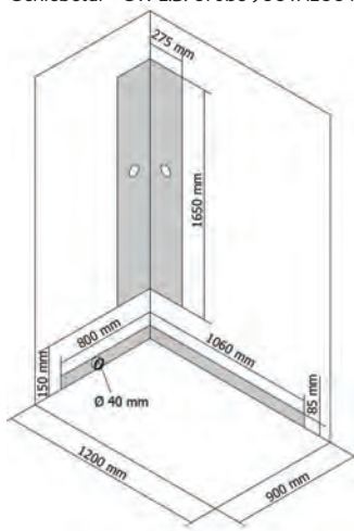
Schiebetür + SW z.B. Größe 900 x 1200 mm
