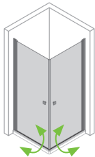
TYP 5333 EckEinstieg Drehtür 2-teilig (5 mm ESG)
